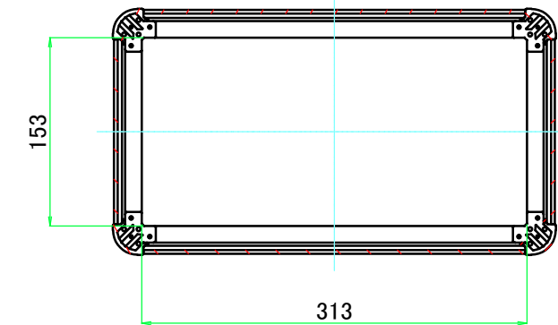
C-C ( 1 : 5.5 )
