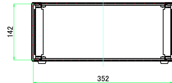
B-B ( 1 : 5.5 )
